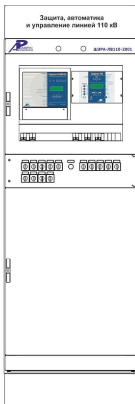
Шкаф защит и АУВ линии 110(220) кВ ШЭРА-ЛВ110-2001 БПВА.656457.054, БПВА.650645.001 ТУ
